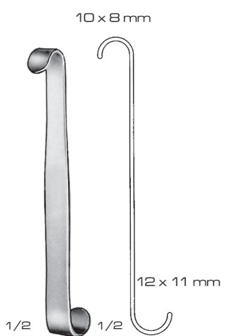
Luer 03-890-11 11 cm / 4¼"
